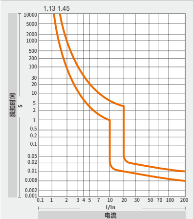
D曲线
